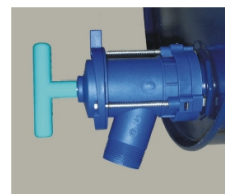
Fatkran Art.nr. Tappo för det stora sprundet 2" fästes med ett enkelt handgrepp. Med kranens T-handtag lossas befintligt fatlock, vätska tappas och fatlocket återmonteras .
